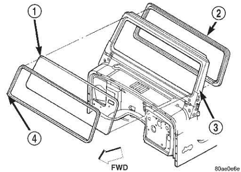
Fig. 2 Windshield
